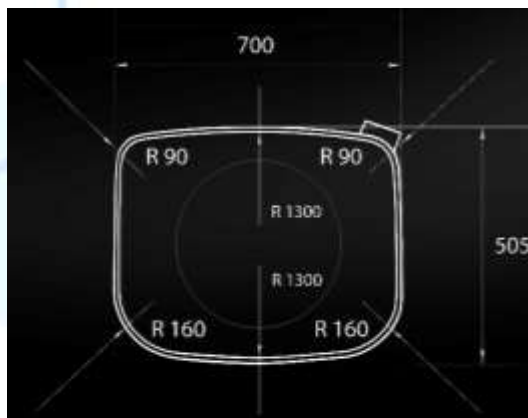
2-rasm. Yuk avtomobili yoqilg'i baki qismlarining gabarit o'lchamlari sxemasi
