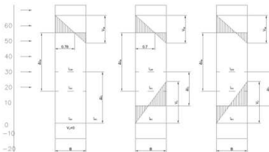
Рис. 1.4 Изменения средних температур \Delta t_w и \Delta t_c – бетона и перепады температур \vartheta_w , \vartheta_c по сечению стению стены из бетона в жаркое и холодное время года;
