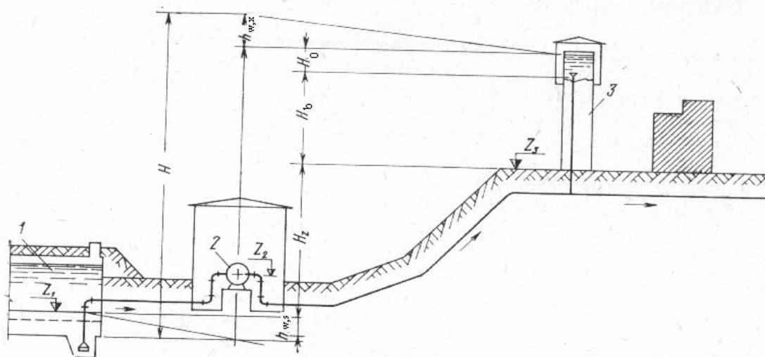
2-rasm. Suv ta'minoti tizimidagi ikkinchi ko'taruv nasos stantsiya tasviri: 1-toza suv havzasi (idishi); 2-nasos; 3-suv minorasi
