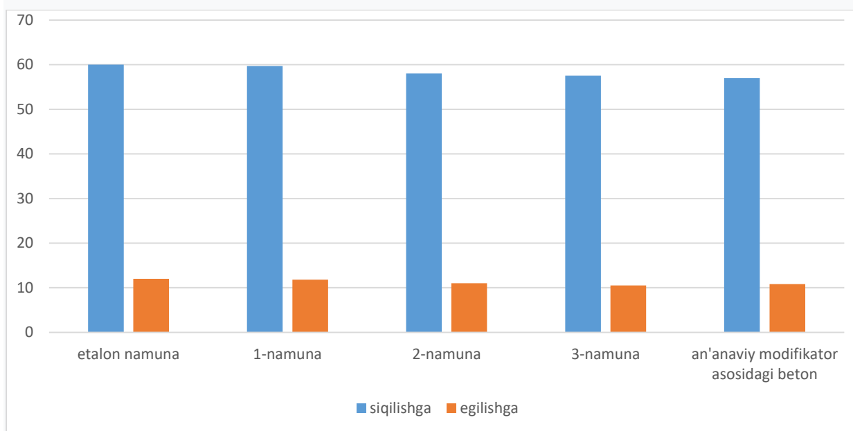
1-расм. Модификатор қўшилган намуналар ва анъанавий модификатор асосидаги олтингугурт бетоннинг мустаҳкамлик кўрсаткичалари диаграммаси.
