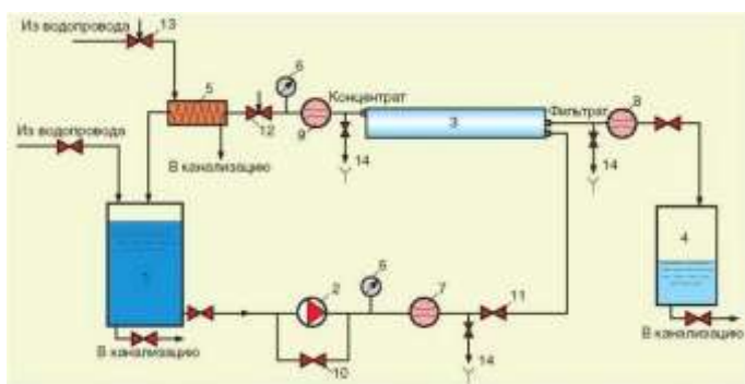
Рис. 3. Схема экспериментальной установки очистки воды с нанофильтрационными и обратноосмотическими мембранами:
