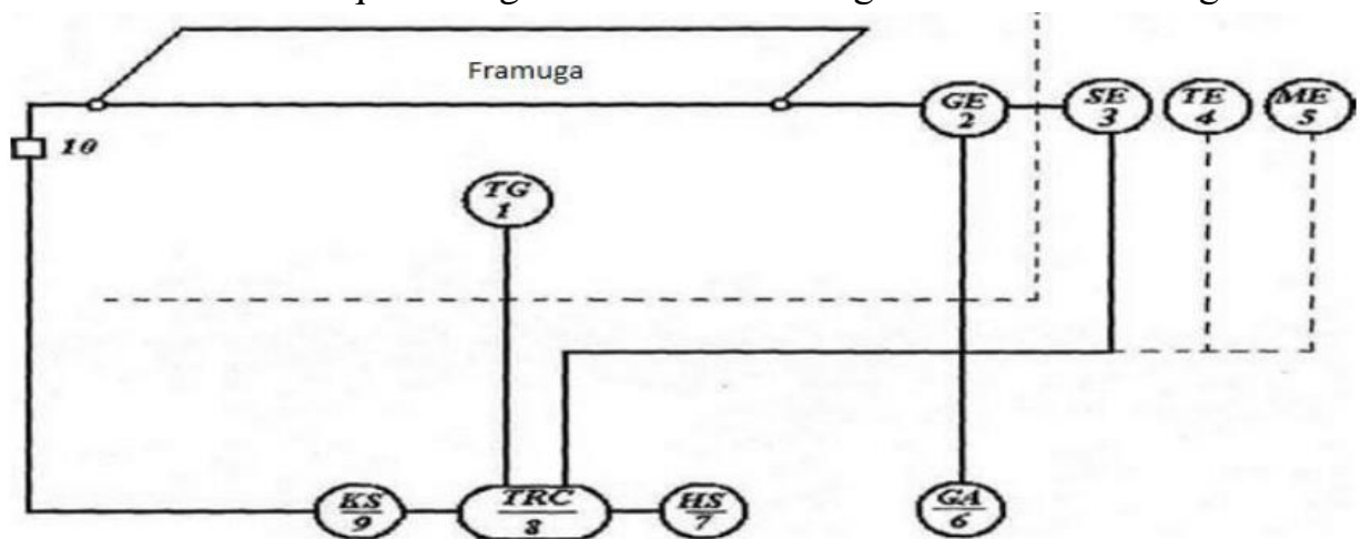
4-Sxemada Issiqxonada tabiiy ventilatsiyani boshqarish funksional - texnologik sxemasi.
