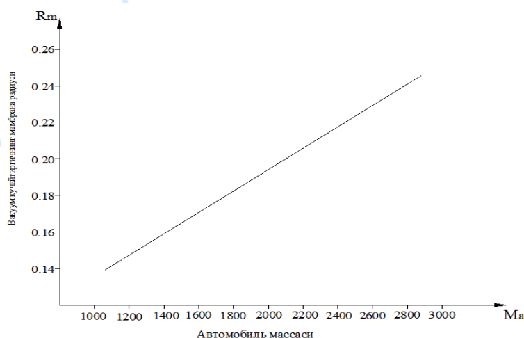
2.2-rasm. Vakuum kuchaytirgich membranasi radiusini avtomobil massasiga bog‘liqlik grafigi.
