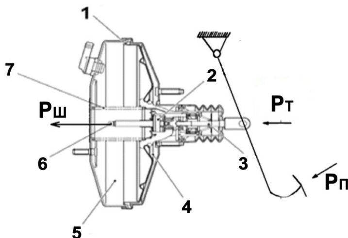
1-rasm. Vakuum kuchaytirgichni hisoblash sxemasi.
