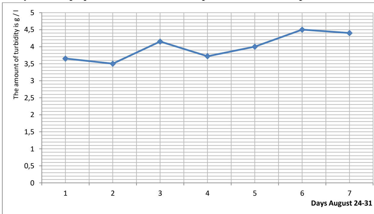
Рис. 2. Изменение количества мутности в структуре стока в долине реки Сохсай.
