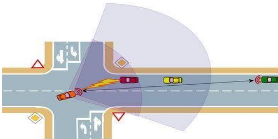
4-rasm - Burilish paytida yordam tizimining ishlash sxemasi.
